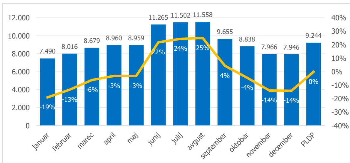
Dnevne obremenitve po mesecih za leto 2019, AŠM 650 Ankaran
