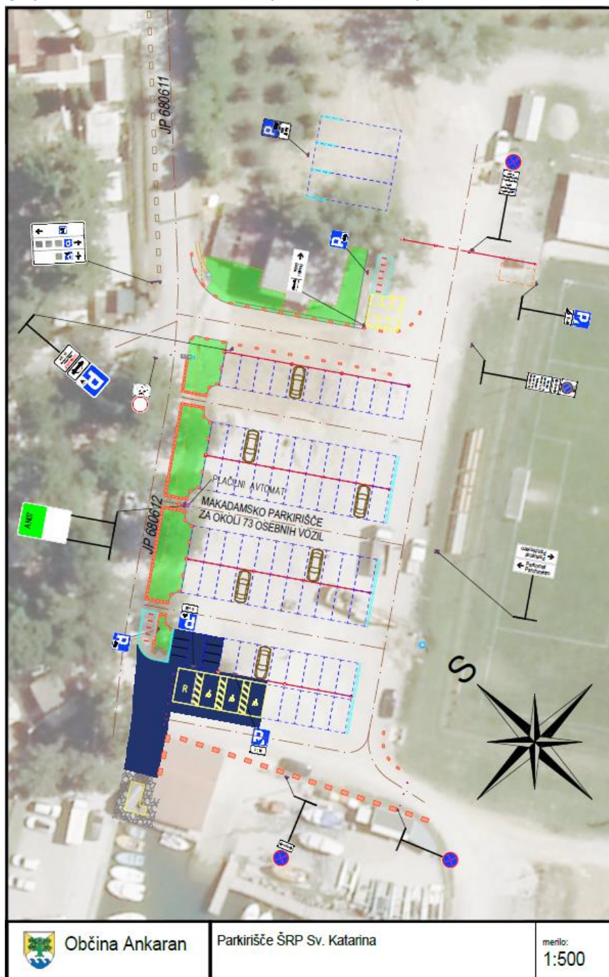
Slika: Načrt javnega parkirišča ŠRP Sv. Katarina s prikazanimi tremi parkirnimi mesti za avtobuse.
