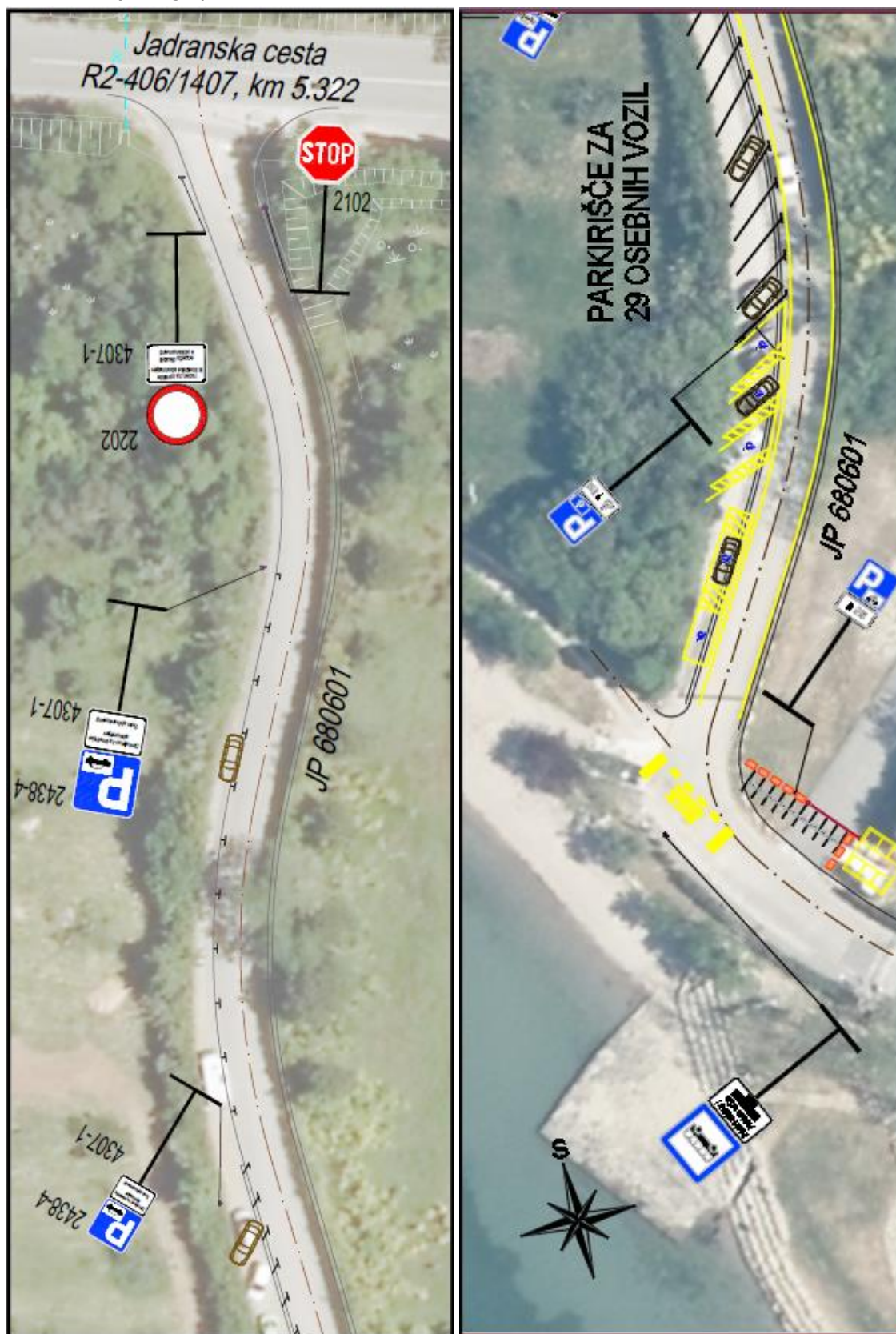
Slika: Načrt javnega parkirišča Valdoltra - zahod.
