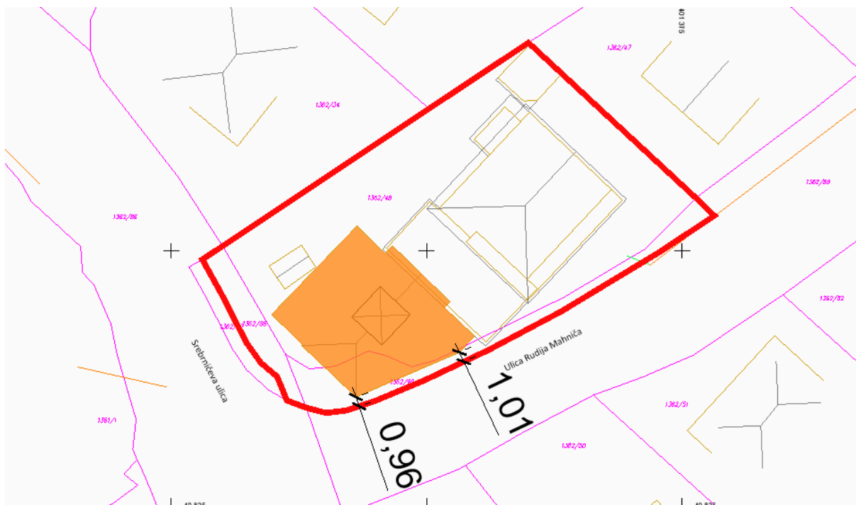
Slika 6: Izsek iz geodetskega načrta s prikazom najmanjših odmikov nadstreška od parcelne meje
